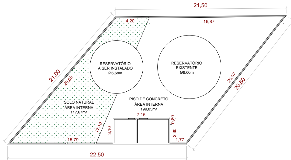
Figura 01 – Croqui do terreno onde será instalado o reservatório
